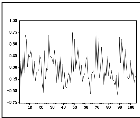
Gráfico 1: Residuos de la función de costos, firma típica.
